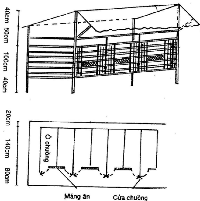
Hình 9 - Chuồng nuôi dê- nhìn tổng thể và mặt bằng
