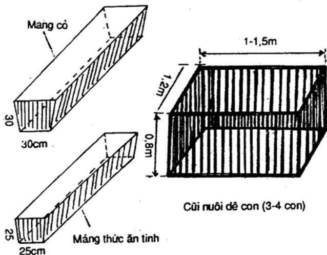
Hình 10 - Yêu cầu kích thước chuồng nuôi, máng ăn, máng uống và cũi dê con
